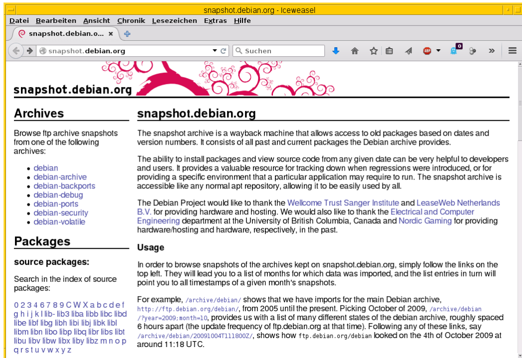
Abbildung 8.30: Das Debian-Paketarchiv
