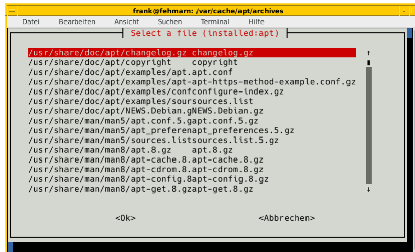
Abbildung 8.23: Aufruf von debman für das Paket apt
